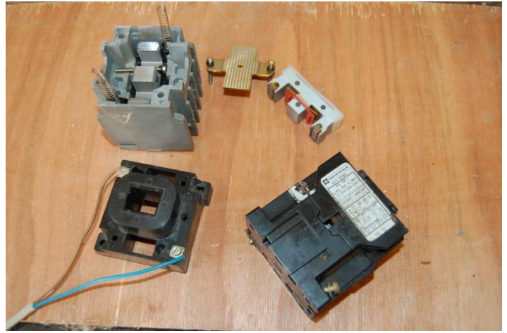
Photo. Un contacteur explosé et un autre entier.
